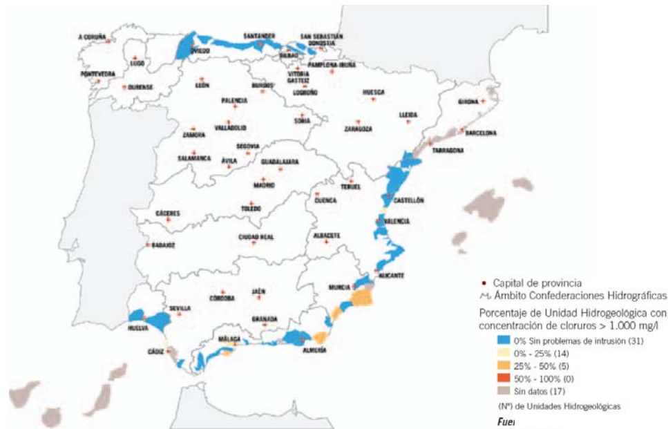
Figura 3. Porcentaje de superficie de unidad hidrogeológica costera con concentración de cloruros > 1.000 mg/l (2003) (Fte. Perfil Ambiental de España 2005)
